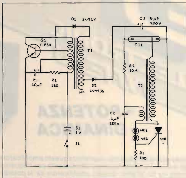
figura 10 Lo schema del lampeggiatore di fig. 8.
