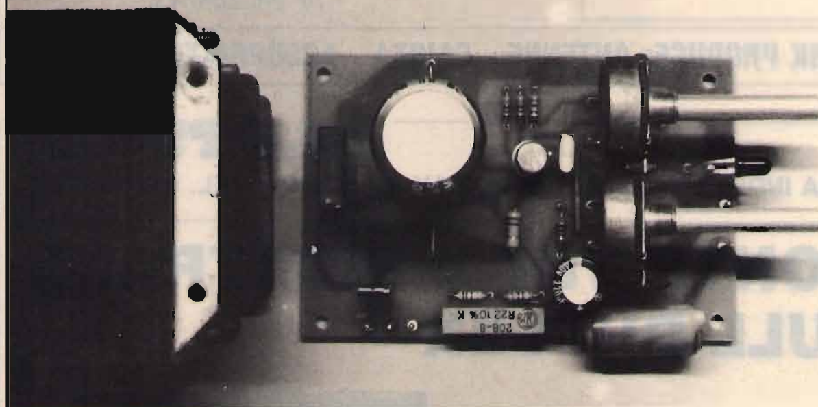
figura 4 Un esemplare dell'alimentatore stabilizzato al termine delle operazioni di montaggio.
