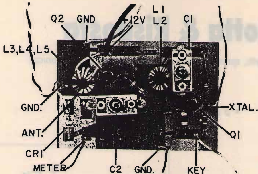
figura 3 Un prototipo del trasmettitore-pilota da 1 watt illustrante la disposizione dei componenti sul circuito stampato.
