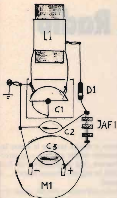
figura 2 Piano di cablaggio dell'ondametro ad assorbimento.
