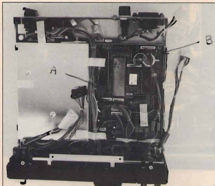
foto 3 Le frecce indicano: A) il diodo D27; B) i diodi D43 e D44.
