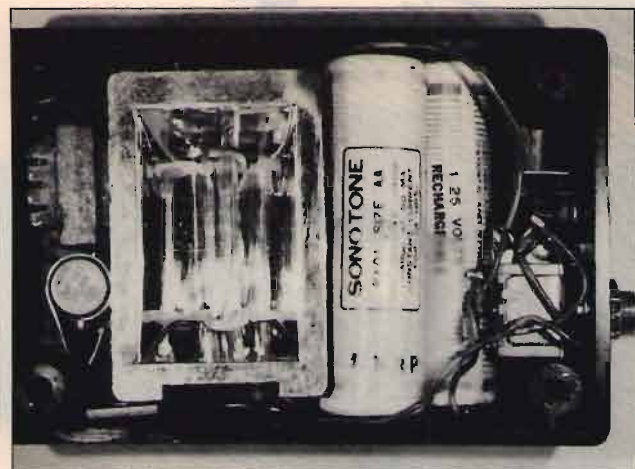
figura 9 L'interno del dispositivo di fig. 8.
