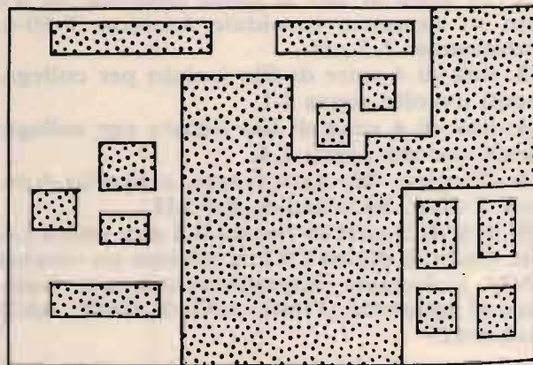
figura 2 Circuito stampato, in grandezza naturale, del trasmettitore-pilota.
