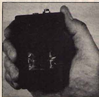
figura 8 Un piccolo lampeggiatore stroboscopico autocostruito impiegando componenti di recupero.
