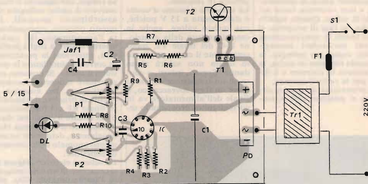
figura 3 Piano di montaggio dell'alimentatore stabilizzato.
