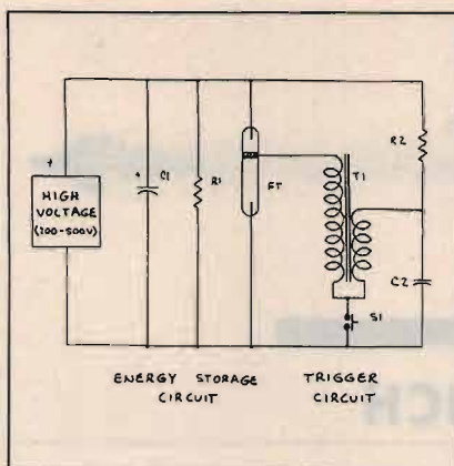
figura 2 Schema di un semplice lampeggiatore. Energy storage circuit = circuito di immagazzinamento dell'energia; trigger circuit = circuito di innesco.
