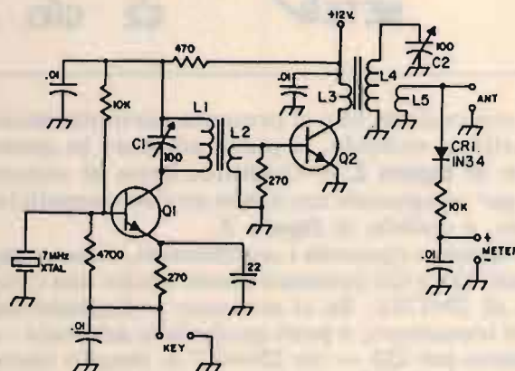
figura 1 Schema elettrico di un trasmettitore-pilota in grado di erogare la potenza di 1 watt a 21 MHz.
