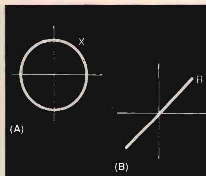
figura 9 Ellisse di Lissajous per una reattanza puramente capacitiva (A) e per una resistenza pura (B).
