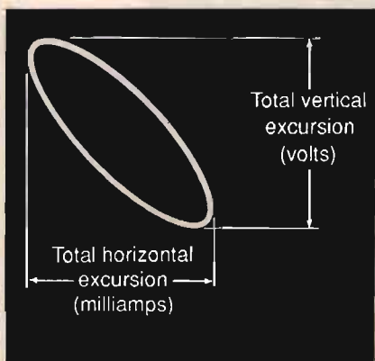
figura 10 Il rapporto tra escursioni totali verticale e orizzontale dell'ellisse di Lissajous fornisce una misura dell'impedenza.
