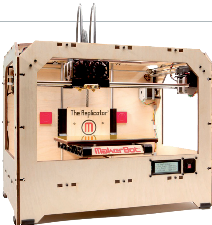
Fig. 8 Makerbot Replicator è la stampante che dalla primavera 2012 viene venduta da Makerbot Industries, in kit a circa 1700 dollari.
