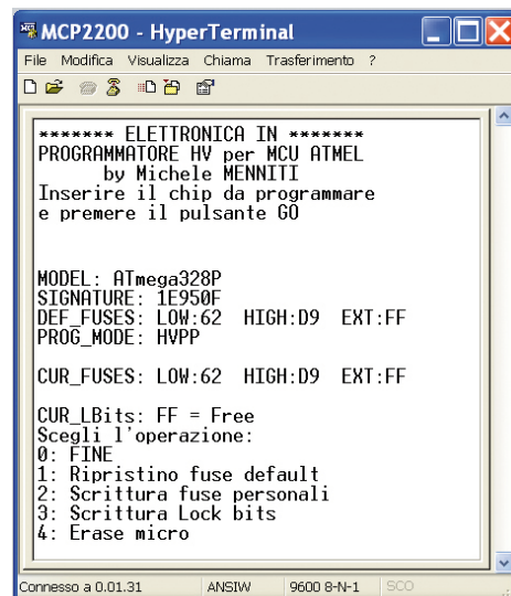
Fig. 5 - La schermata iniziale del firmware PC su HyperTerminal
