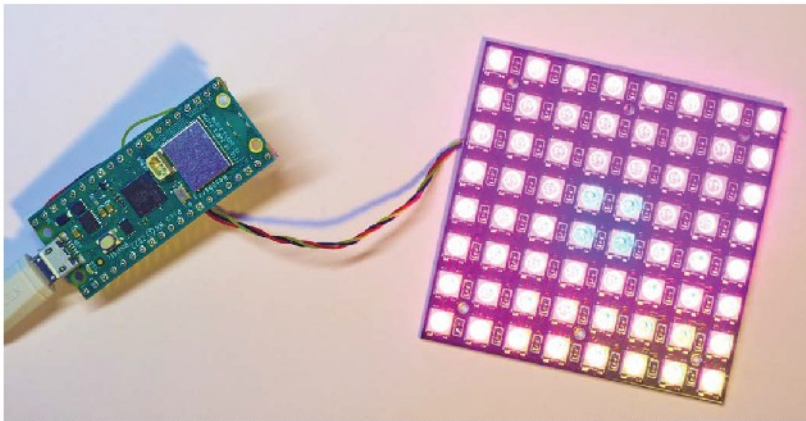
◀ Figura 3: Il pannello è collegato ai pin VSYS, GND e GPIO18 di Pico
