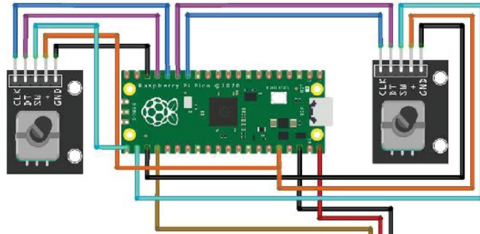
◀ Figura 2: Lo schema elettrico del progetto
