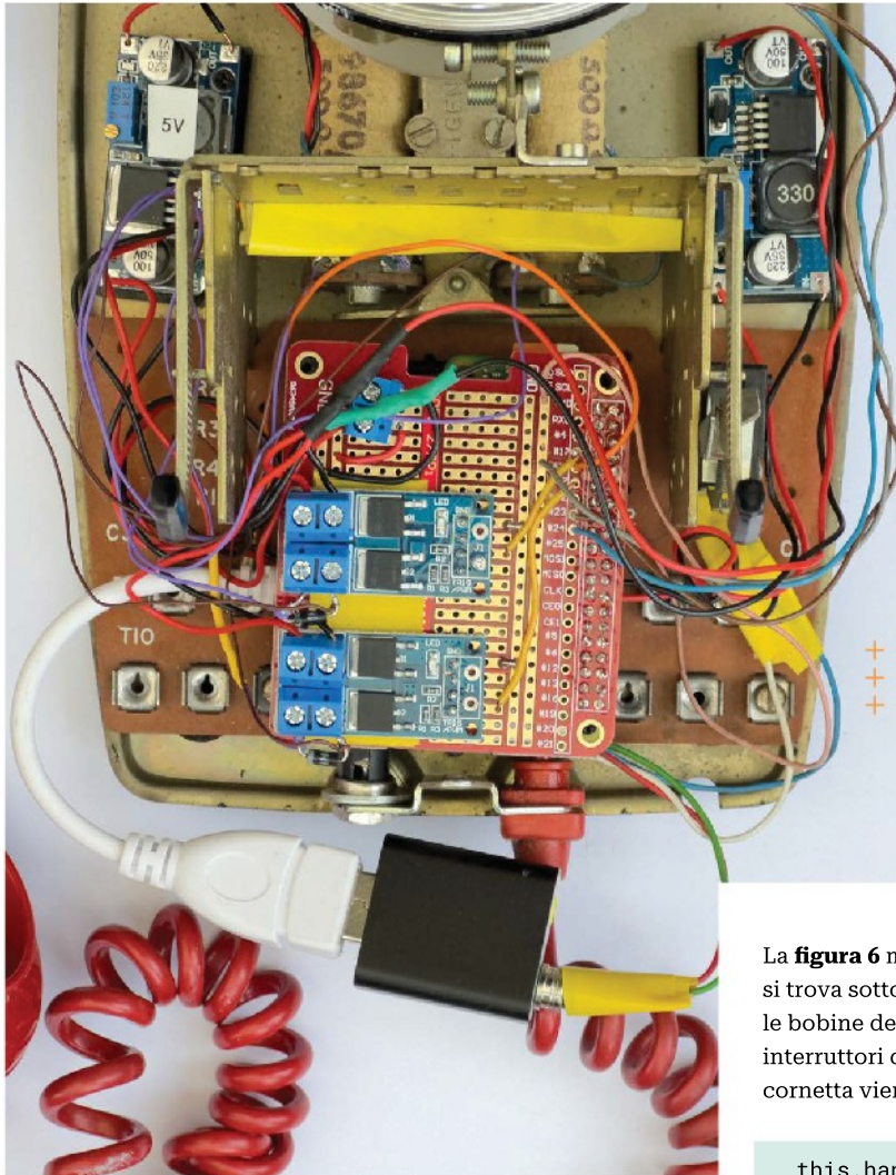
◀ Figura 6: Un'interfaccia audio USB è collegata all'altoparlante del telefono.
