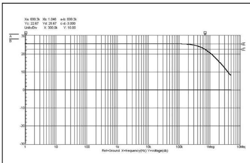
Fig. 7 - Curva di risposta in frequenza dello stadio amplificatore con op-amp di cui alla figura 2 a.
