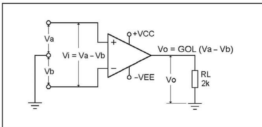
Fig. 3 - L'amplificazione è sempre data dal rapporto fra il segnale di uscita V_o e la differenza (V_a - V_b) = V_i dei segnali applicati ai due ingressi. Se uno dei due ingressi è a massa, per esempio l'ingresso b , allora V_b = 0 e quindi V_i = V_a . Il guadagno sarà allora fornito dal rapporto V_o/V_i = V_o/V_a .
