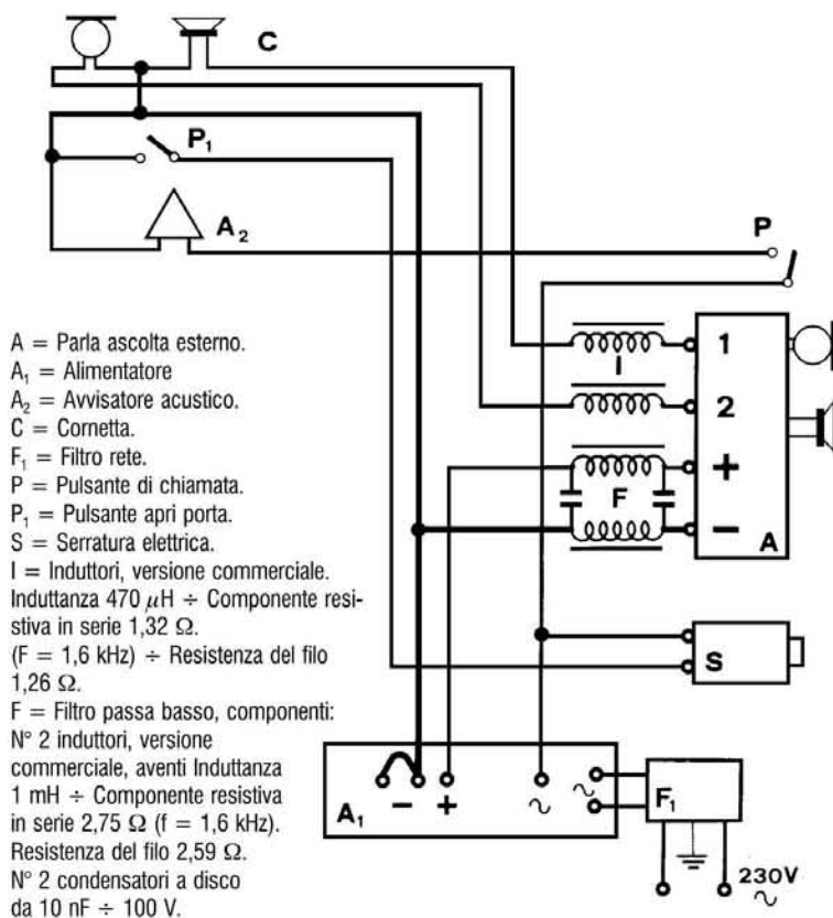
Fig. 5 - Citofono, schema di principio
