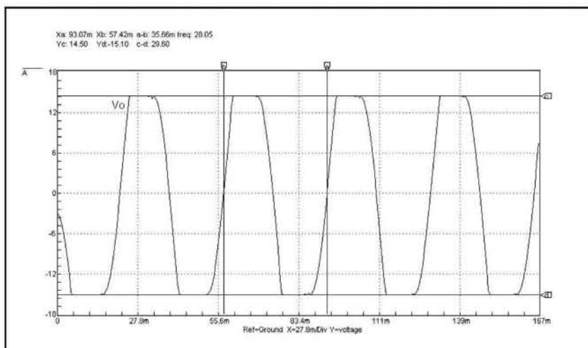
Fig. 5 - Usando l'op-amp ad anello aperto basta un segnale di ingresso di pochi microvolt per portare l'uscita in saturazione.
