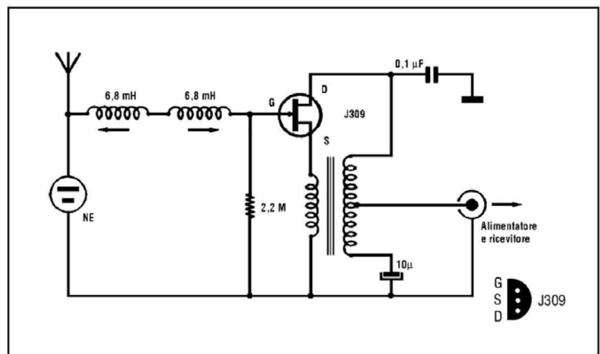
Fig. 3 - Il trasformatore è un vecchio intertransistoriale. Il J309 deve essere selezionato per una corrente di funzionamento di 12 \div 16 mA. Eventualmente ridurla con un gruppo R-C sul source con C \leq 1000 \mu F .
