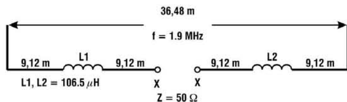
Fig. 1 - Sistema per adattare un dipolo per gli 80 m sui 160.
