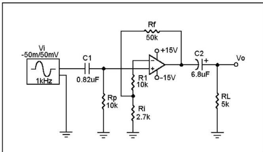
Fig. 9 - La resistenza R_i svincola il valore della resistenza R_p - che fissa la resistenza di ingresso dello stadio - dai valori attribuiti alle resistenze R_f e R_i .
