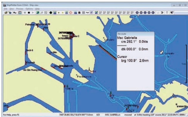
Ricezione del protocollo Automatic Identification System (AIS) con ShipPlotter - circa 20 navi individuate a Porto Marghera
