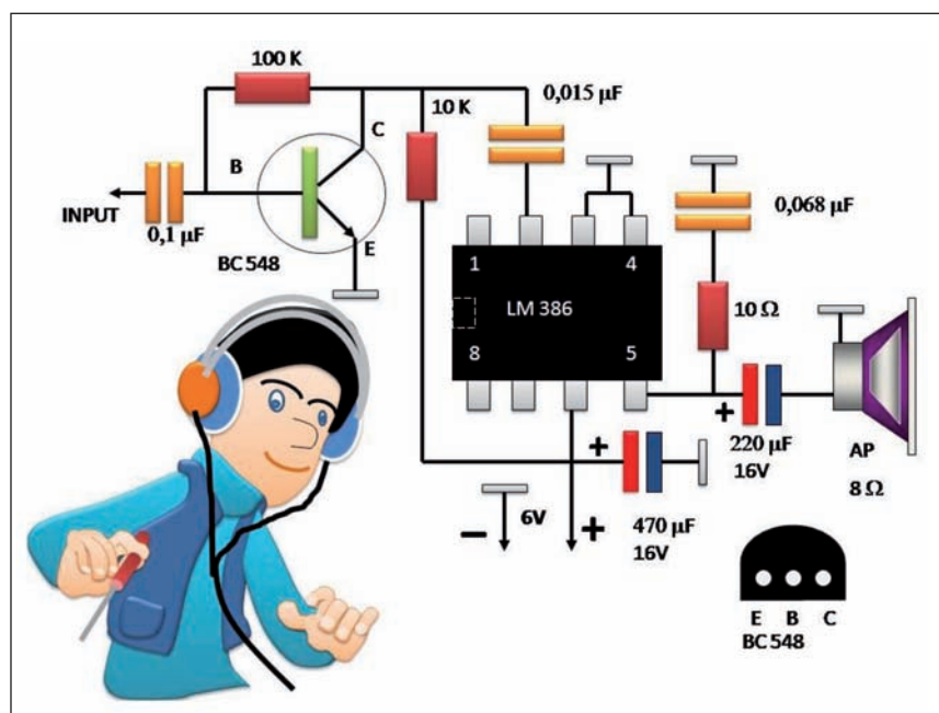
Schema elettrico dell'amplificatore audio realizzato con l'IC LM 386
