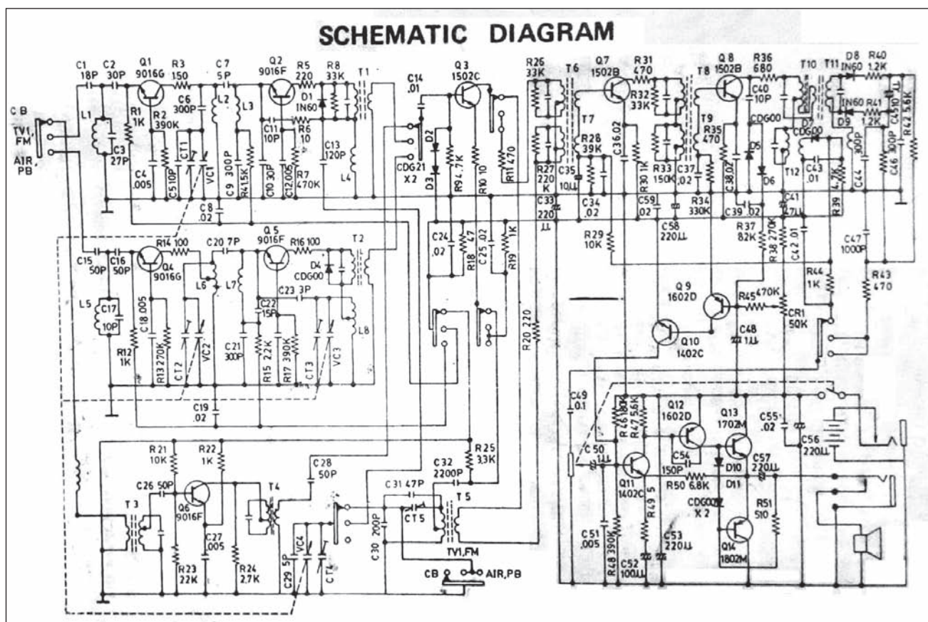
Schema elettrico del ricevitore radio Lafayette TR 80.
