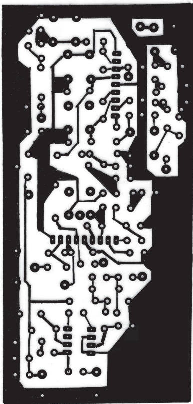
Fig. 2 - Circuito stampato lato rame
