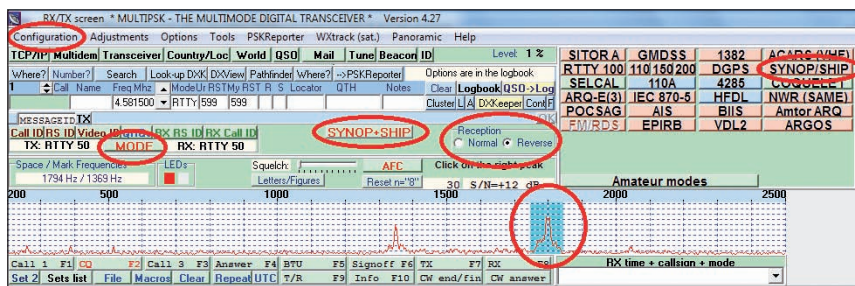
Fig 4 - MULTIPSK
