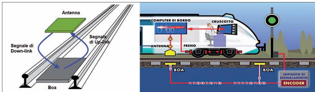
Fig. 2 - A sinistra lo schema base che illustra l'operatività del sistema, a destra l'applicazione nella forma più completa dove le boe sono interconnesse con gli impianti di segnalamento.
