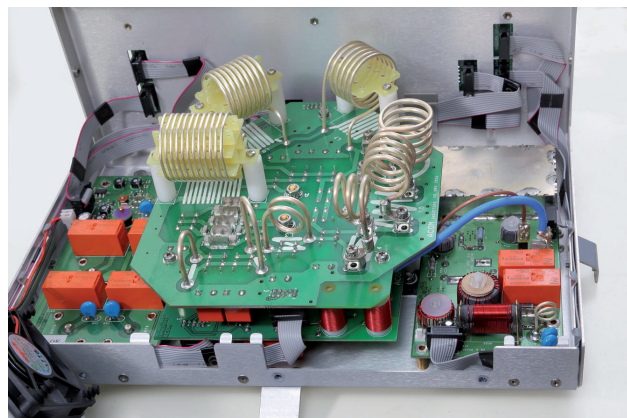
Fig. 11 - 04AT interno.
