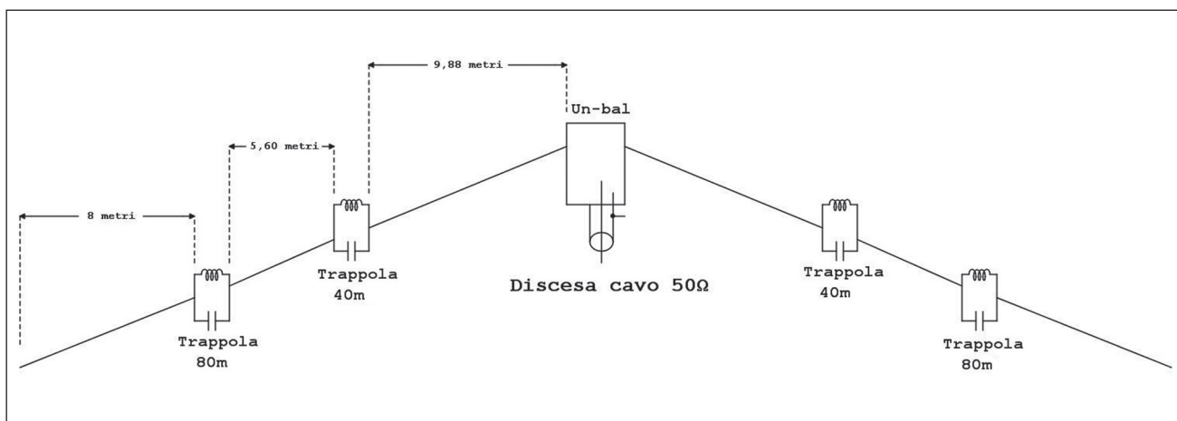
Fig. 1 - Schema dipolo
