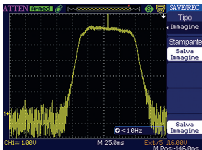
Fig. 7 - Curva di risposta di un filtro a 11 MHz, scansione 1 kHz/div.
