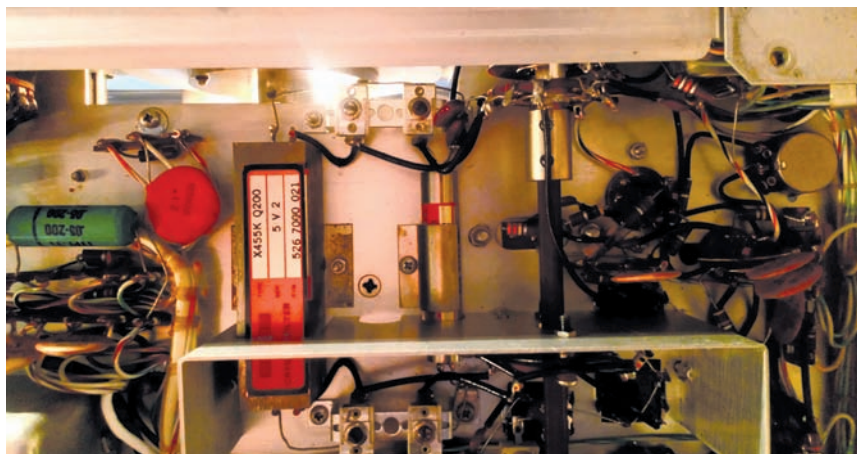
Foto 2 - Filtro a cristallo Collins tipo X455K Q200.
