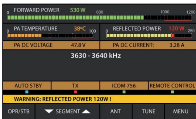
Fig. 14 - Display menù principale.
