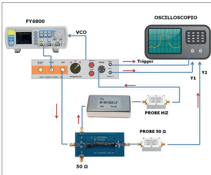
Fig. 9 - Set di misura della funzione di trasferimento e Return Loss
