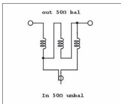
Fig. 2 - Schema 1:1 Un-bal
