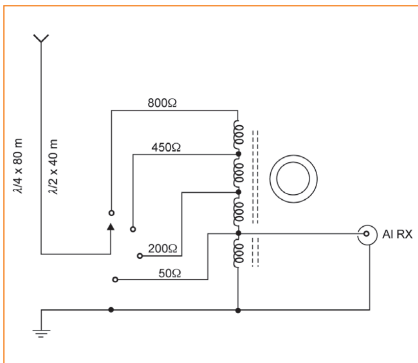
Schema 4 - Adattatore d'antenna
