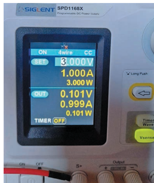
Fig. 2 - Lo strumento sta misurando, senza l'aiuto di un millivoltmetro, una resistenza da 0,1 \Omega . Qui la connessione a quattro fili è d'obbligo. Il calcolo del valore è facile R = V/I = 0,101 / 0,999 = 0,1011 \Omega
