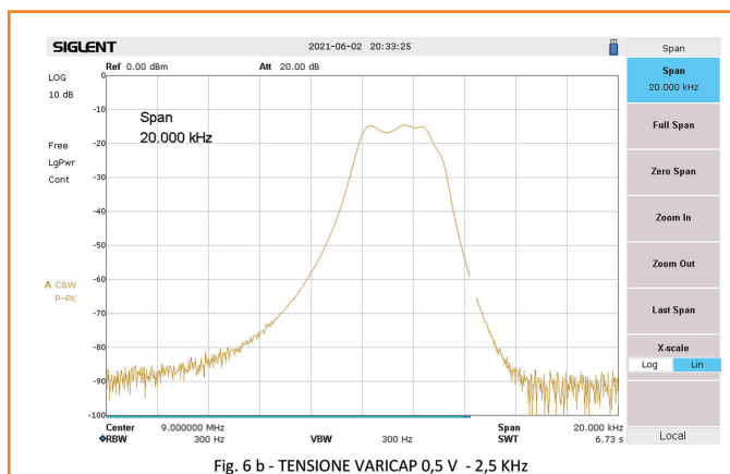
Fig. 6 b - TENSIONE VARICAP 0,5 V - 2,5 KHz
