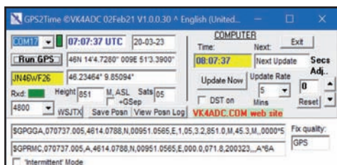
Figura 5 - Programma GPS2Time, di VK4ADC. Questo programma è dedicato alla sincronizzazione esclusivamente via GPS.
