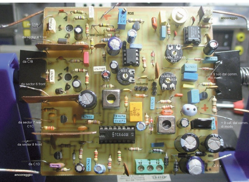
La scheda pronta per l'installazione
