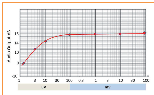
Fig 7 - Risposta AGC
