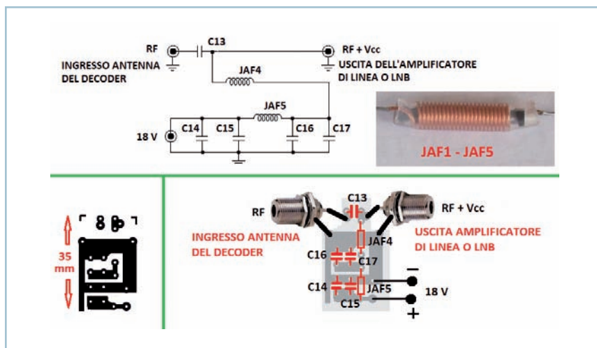
Fig. 9 - L'inseritore di tensione al completo
