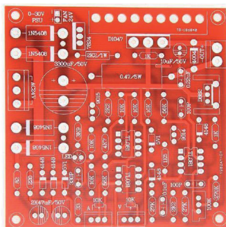
Serigrafia corretta
