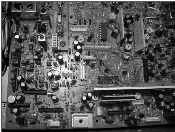
Sotto il coperchio del ricevitore (manopole a sinistra, bocchettoni di antenna a destra) si trova il PCB, qui già epurato delle connessioni, dei pettini e delle viti di tenuta.
