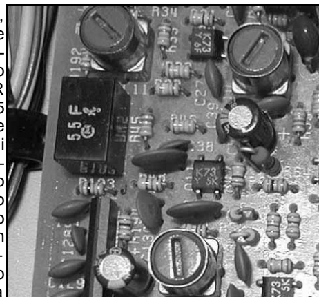
Nel particolare della foto si nota il filtro a 455 kHz (siglato 55 F), la R193, l'IC5.
